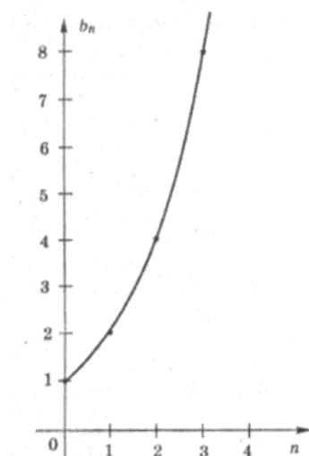
Рисунок 1. Закон, по которому происходит размножение бактерий
